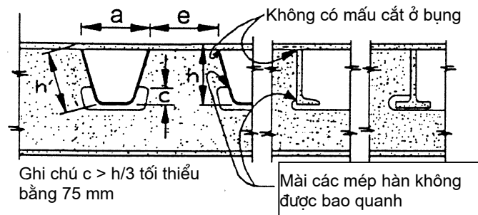
b) Sườn giao nhau với dầm sàn
