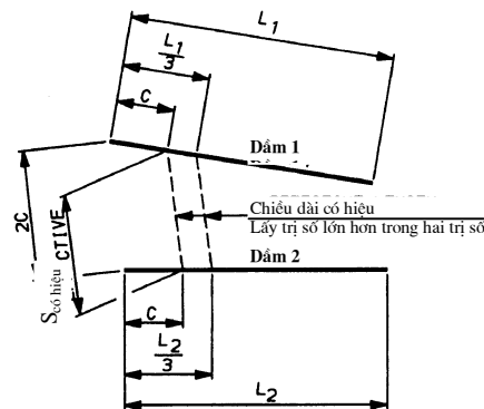
Hình 9.7.2.3-1. Chiều dài hữu hiệu của các dầm cách nhau không đều.
