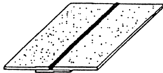
a) Mối nối dọc hàn tại chỗ của bản mặt cầu
